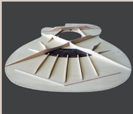
FAN TOP
